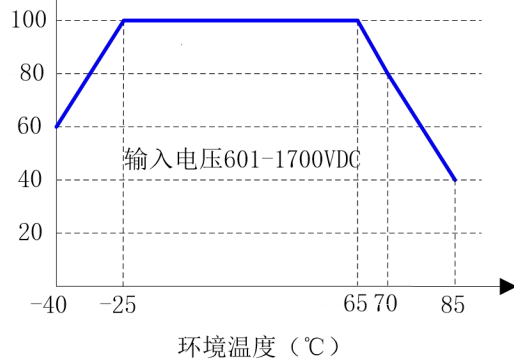
负载随温度降额曲线图A
